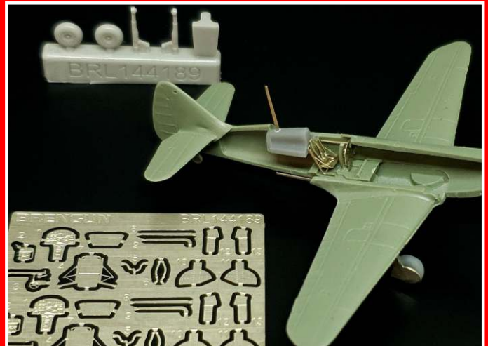
BRL144189 Dewoitine D.520 PE set for Brengun kit
