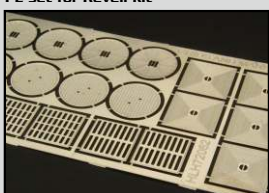
HLH72062 Grills and manholes PE set
