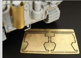
HLU35064 TIGER I Exhaust shroud PE parts for Italeri kit
