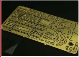
BRL48166 Focke Wulf Ta-154 PE set for Revell kit
