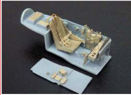
BRL72053 P-38 Lightning pe set for R5 Models kit
