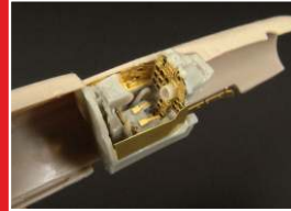
BRL72055 Mig 21 SM/SMT PE set for RV kit
